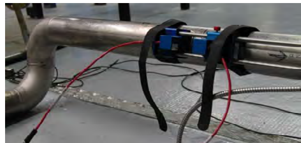
Influence d'un simple coude à 90° (enregistrement)
